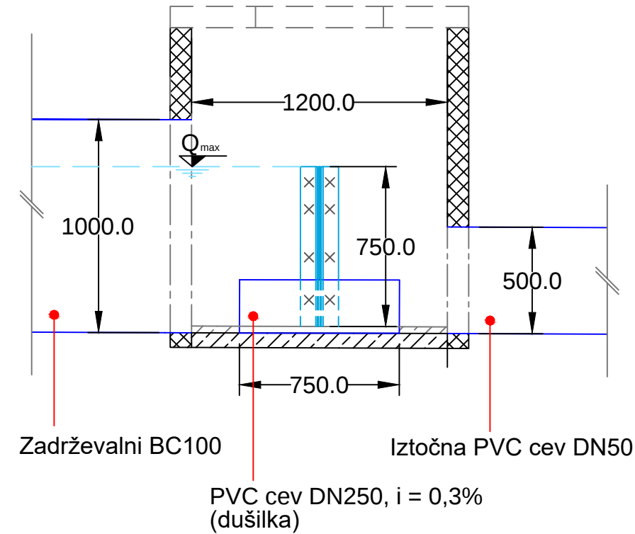
Prerez B-B
